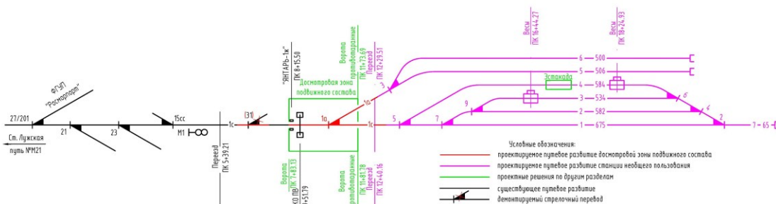
Схема пути необщего пользования ООО «НКТ» после реконструкции приведена на рисунке 3.11.2.
